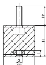
Gummidämpfer / Rubber damper
