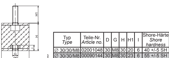
Gummidämpfer / Rubber damper
