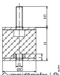
Gummidämpfer / Rubber damper
