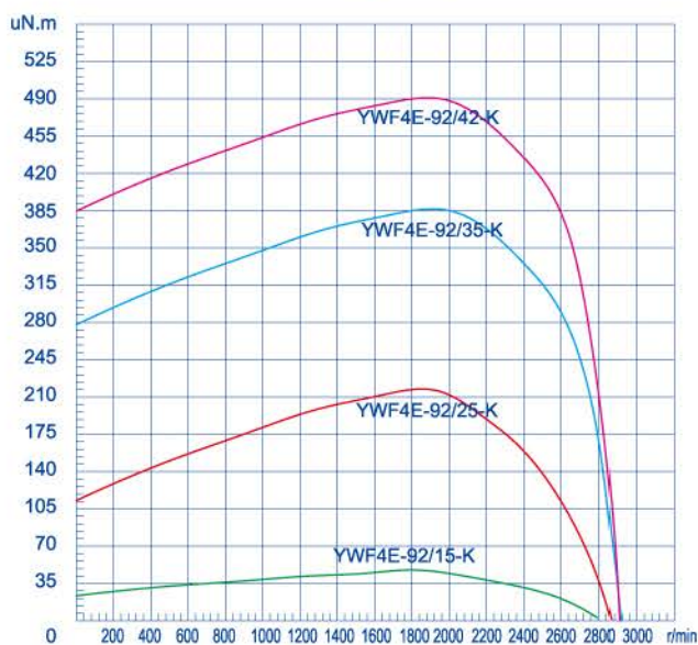
Torque(50Hz)
