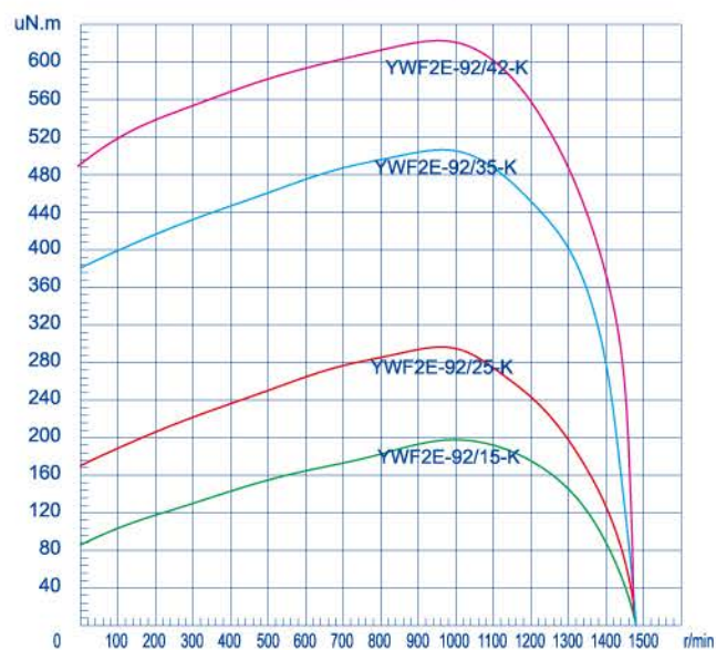
Torque(50Hz)
