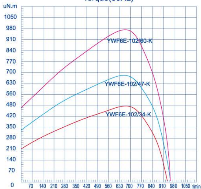
Torque(50Hz)
