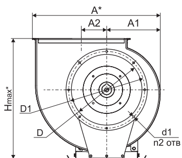
Выходной фланец
