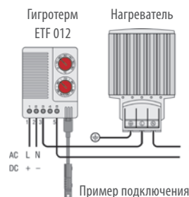
Пример подключения
