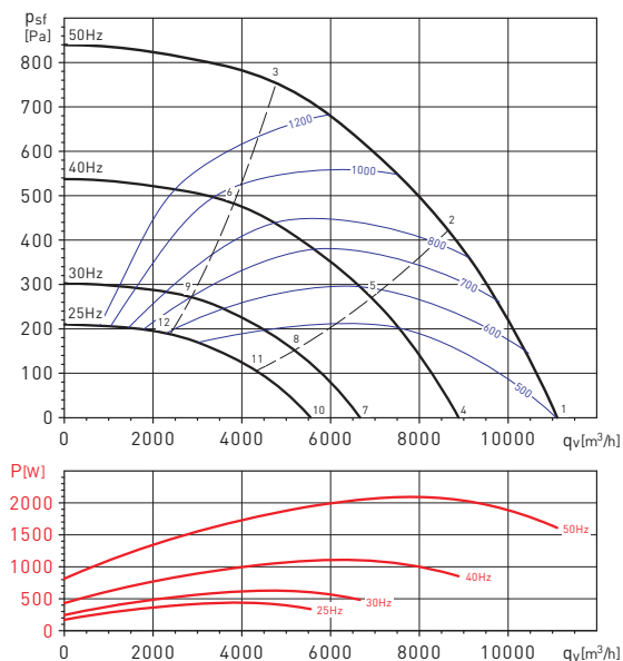
CVAT/4-12000/560N D 2,2kW
