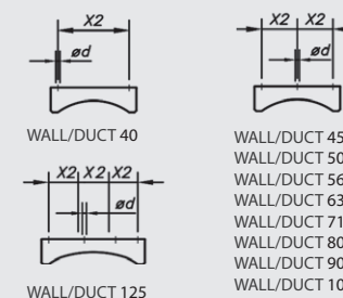
Спиральная опорная стойка
