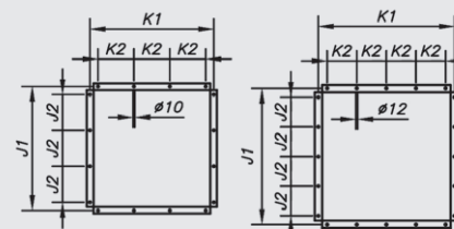
* Фланец для монтажа на стене
