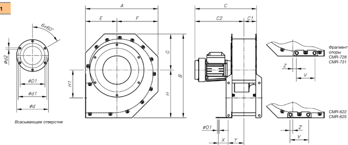
CMRG-622...731
