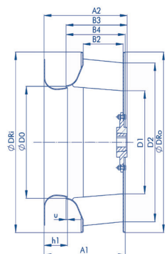
mit Taperlock-Nabe / with Taperlock-Hub
