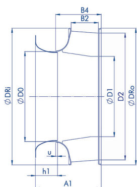
mit Taperlock-Nabe / with Taperlock-Hub
