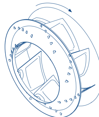
Drehrichtung / Direction of rotation
