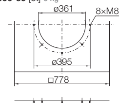
Kabeldurchführung
