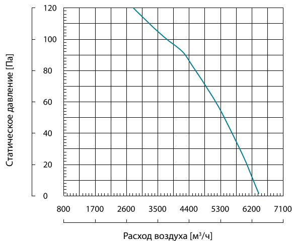
AX-W-500-4E, AX-D-500-4E
