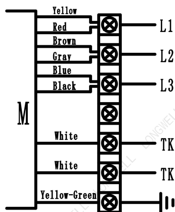
Δ Wiring diagrams
