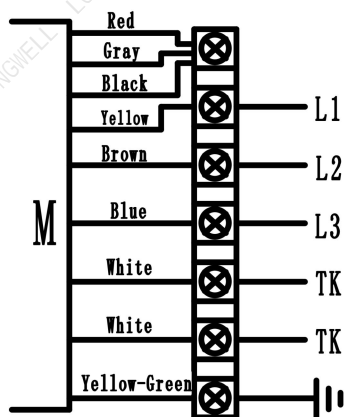
Y Wiring diagrams
