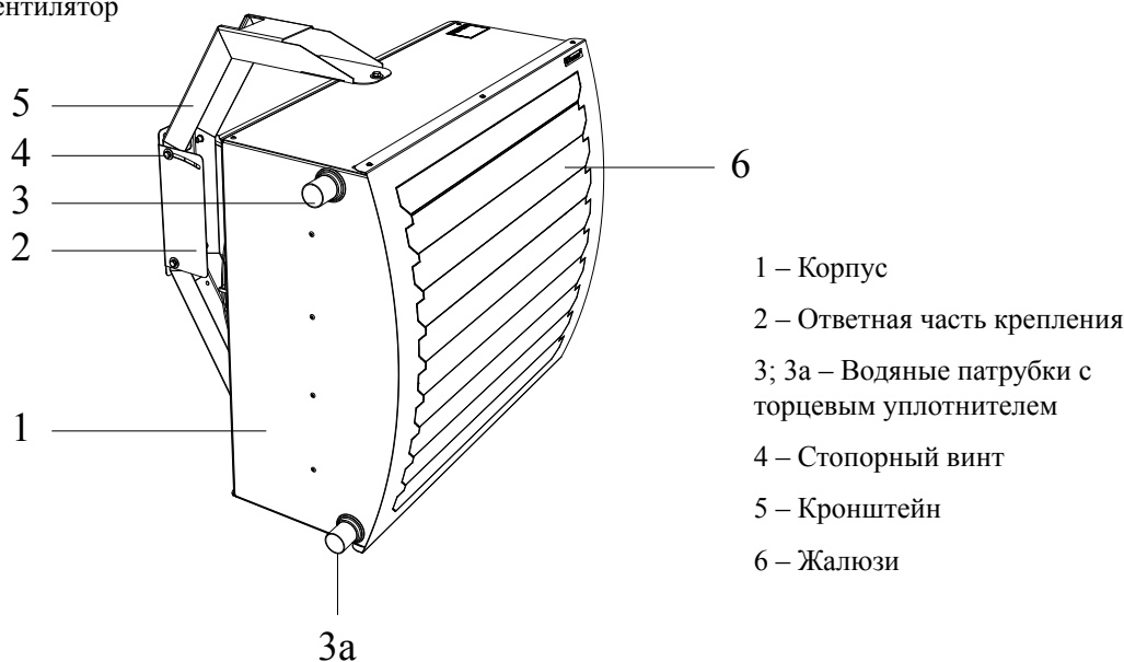
Рисунок 2. Тепловентилятор
