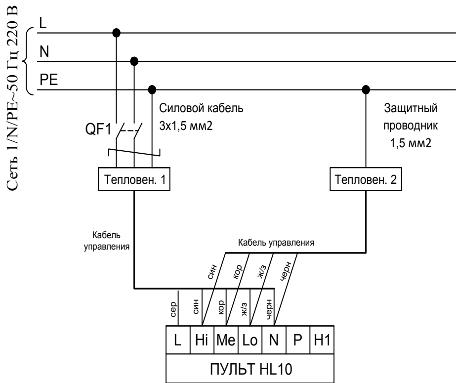
Рисунок 5.1. Схема подключения двух тепловентиляторов к одному пульту управления HL10 с помощью БЛОК-WA.
