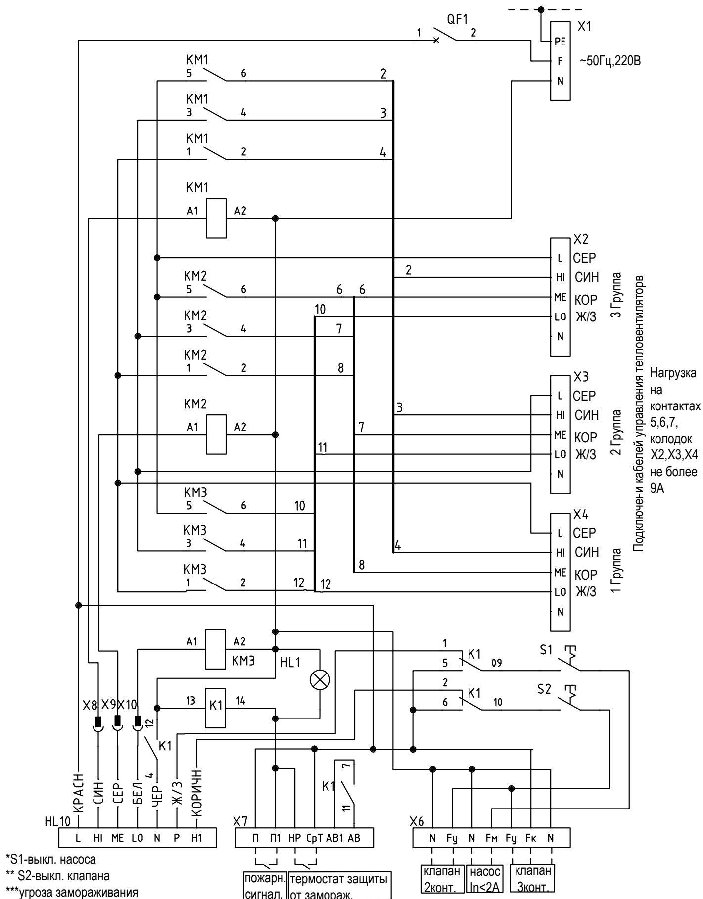
Рисунок 16. Электрическая схема пульта коммутации и управления для тепловентиляторов с водяным источником тепла «ПКУ-W1 (ver 1.0)»
