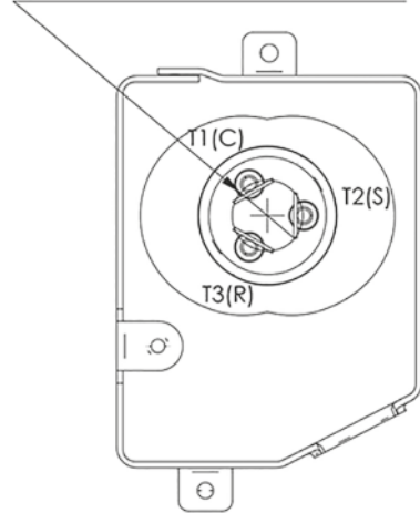
Схема клеммной коробки
