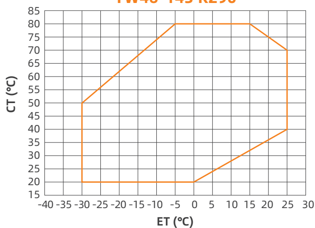
YW46-143 R290
