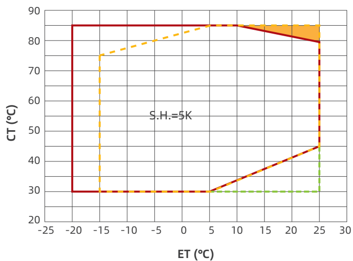
YW38-240/YSW265 R134a
