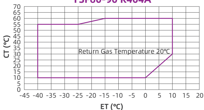
YSF60-90 R404A
