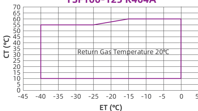
YSF100-125 R404A
