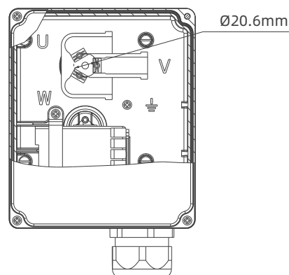
T-Box Layout
