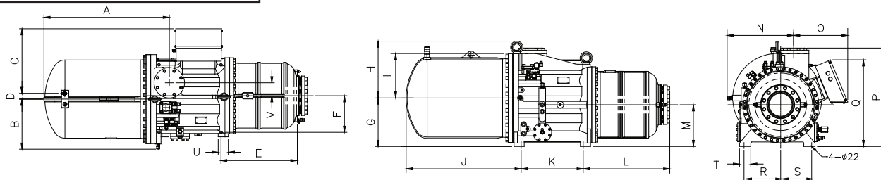
RC2-1020~RC2-1530 Outline
