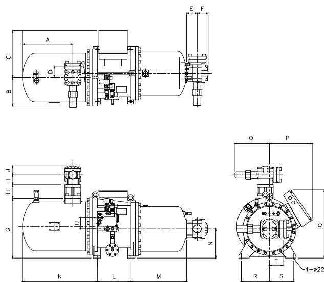
Чертеж RC2-550~RC2-620
