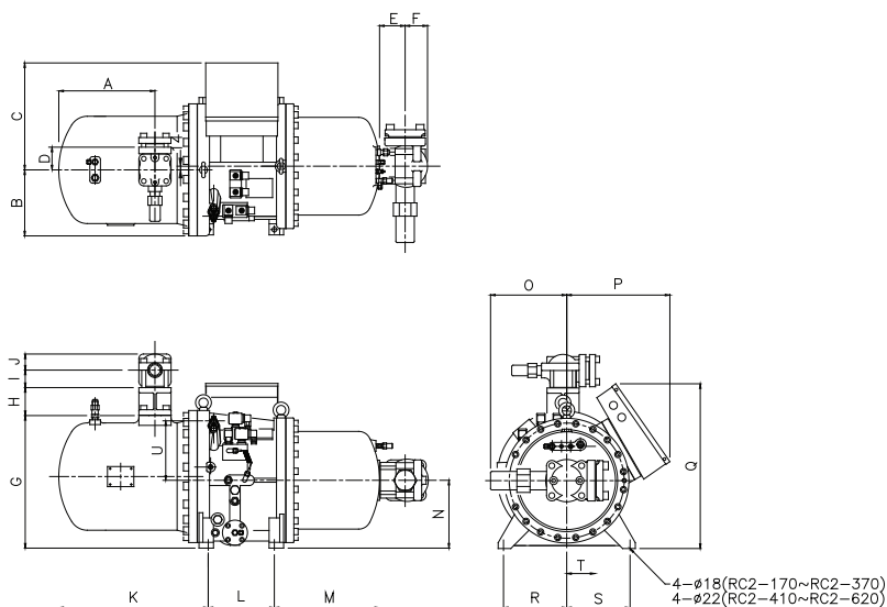
Чертеж RC2-170~RC2-580
