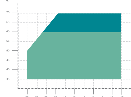
L-M-HBP R134a
