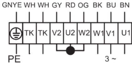
Электрическая схема подключения к вентилятору на 380 - подключение звездой*
