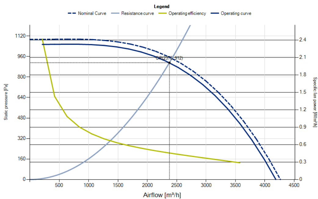
Specific fan power
