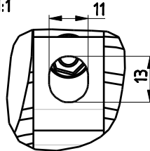
DETALJ 1: 1:1
