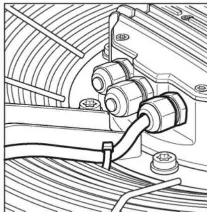
Abb. 3: Liegend eingebauter Ventilator, Verlegung des Kabels als Wassersack.
