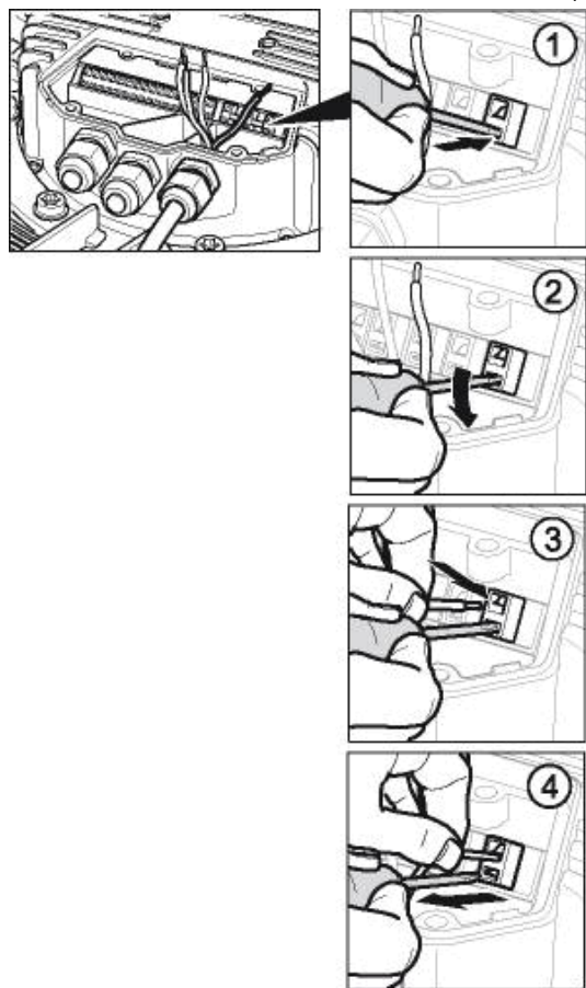
Abb. 2: Anschluss der Leitungen an Klemmen
