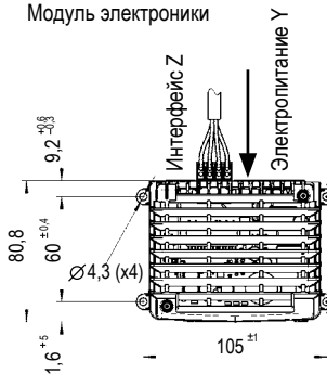
Модуль электроники
