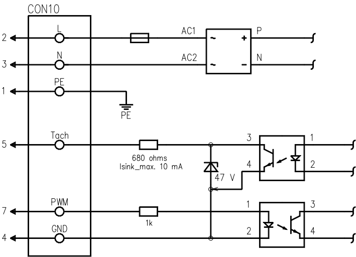
Fan/Motor
