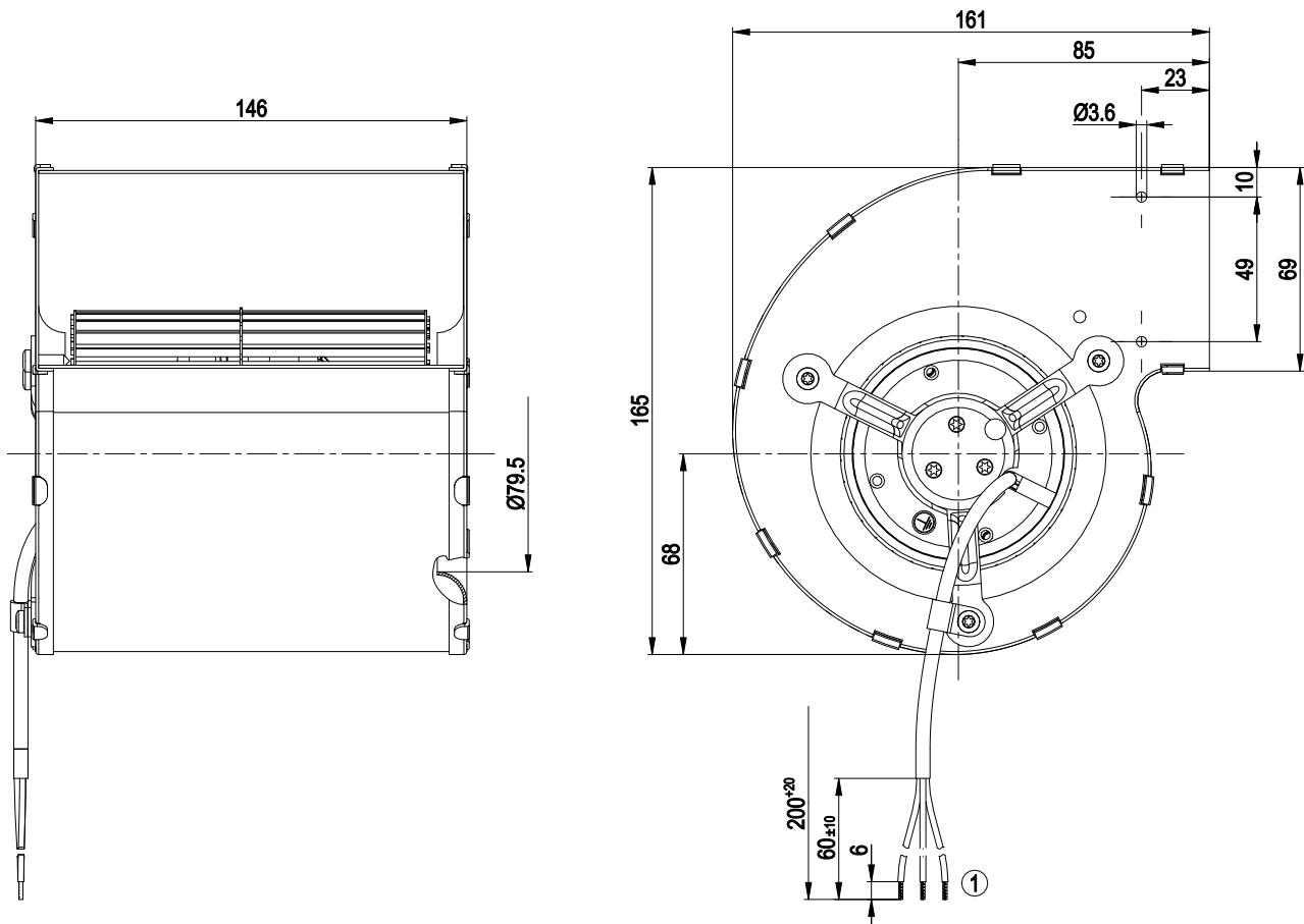
1 Соединительный кабель силиконовый 0,5 мм 2 , 3 присоединенных наконечника для обжима жил
