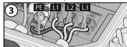
Abb. 2: Anschluss der Leitungen an Klemmen
