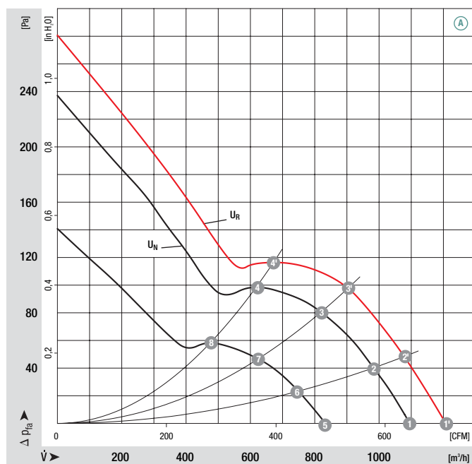
Kennlinien (bei 24 VDC ermittelt)
