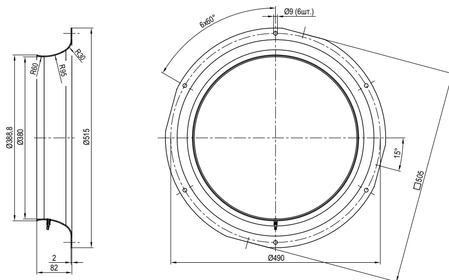
Вентилятор типоразмера 560
