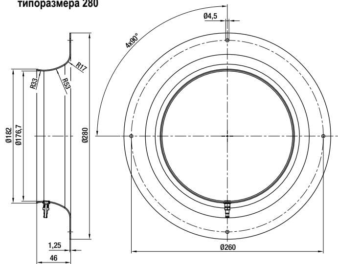
Вентилятор типоразмера 280
