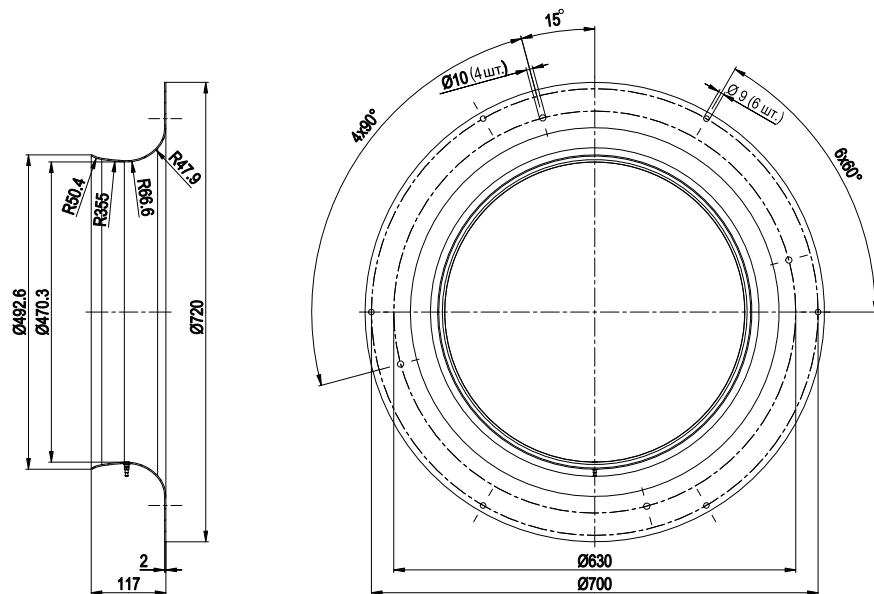
Вентилятор типоразмера 710
