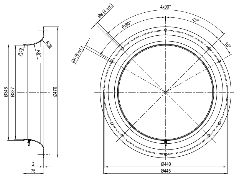
Вентилятор типоразмера 500
