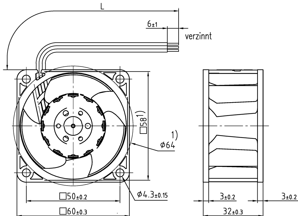
Flanschseite
