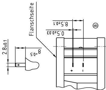
Maße für Steckeranschluß
