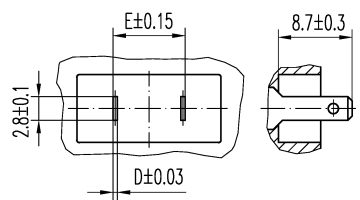
Steckmaße M2:1
