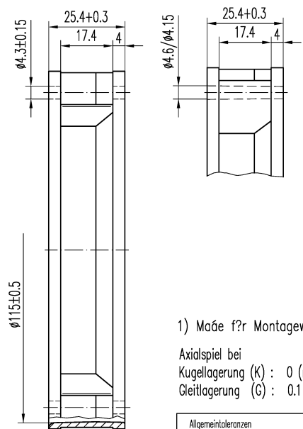
Ausführung F
