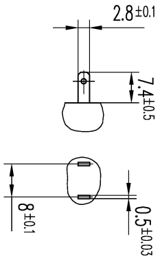
Maße für Steckeranschluß
