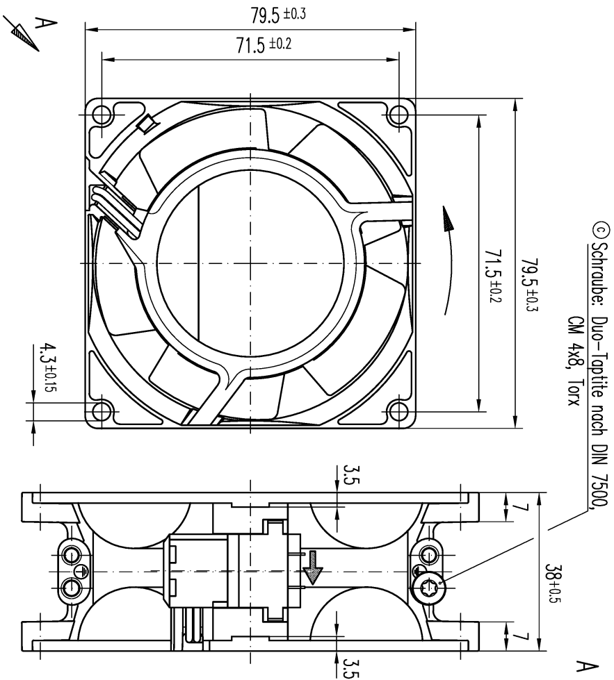
Maße für Steckeranschluß
