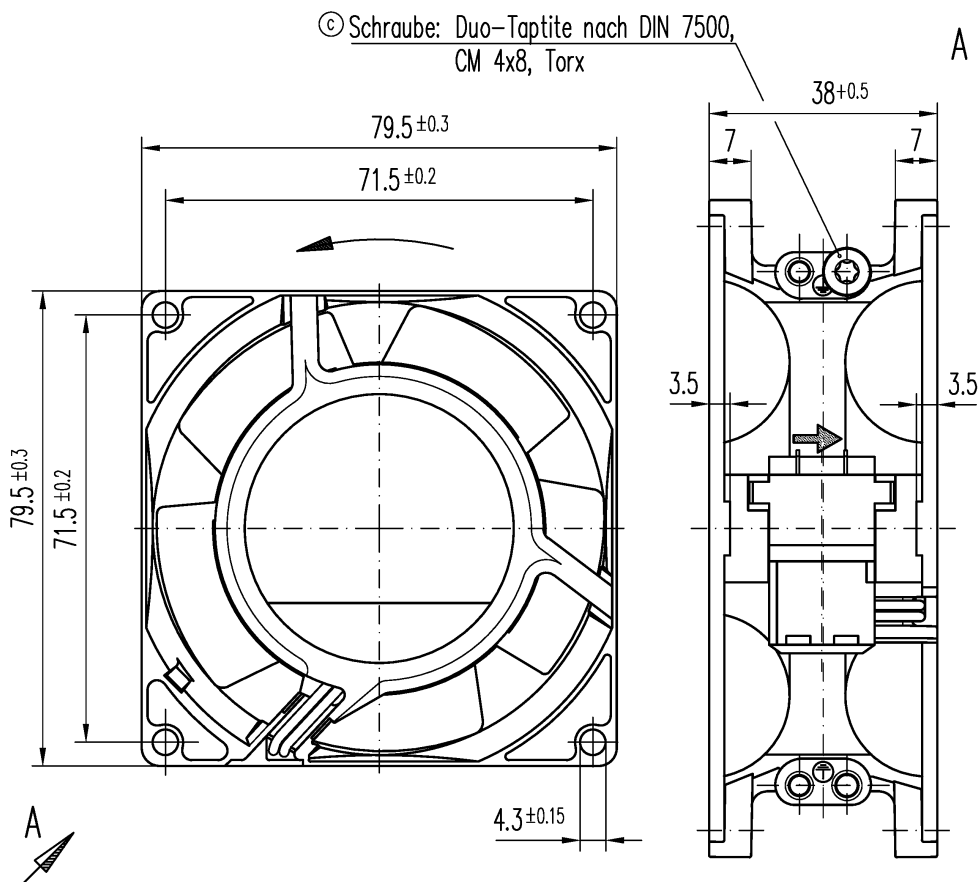
Maße für Montagewand
