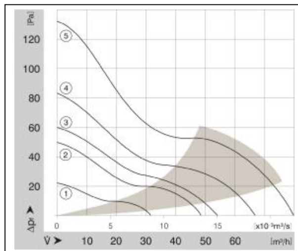
Identische Luftleistungswerte
