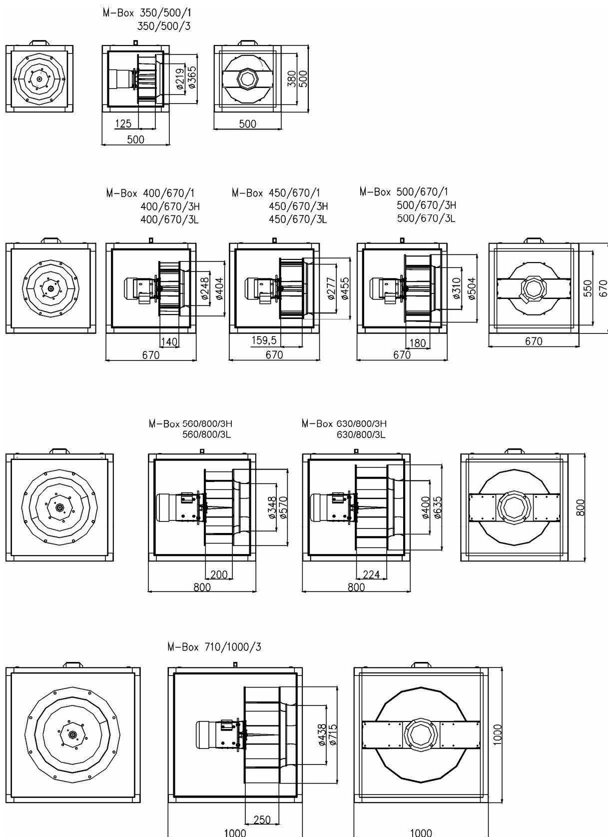
Рис.2 Размеры вентиляторов
