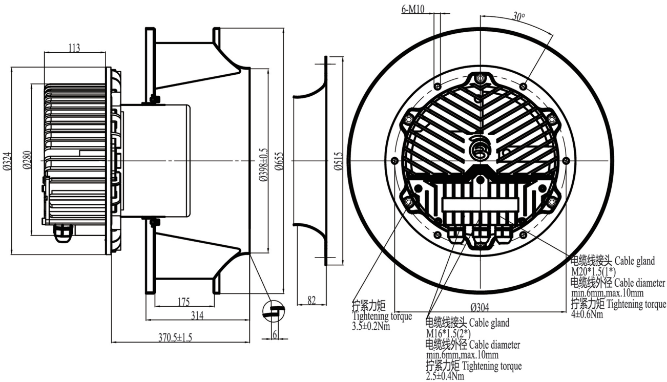
HJ6EC560/188风机整机外形图
