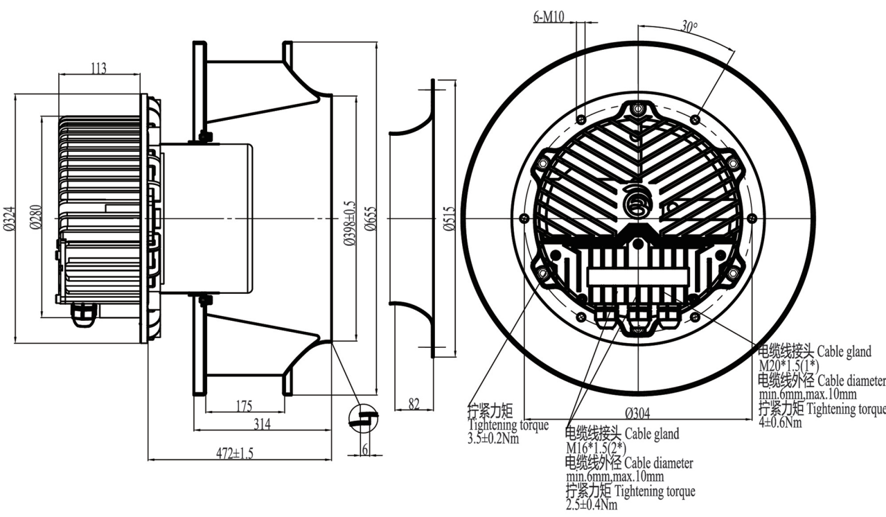
HJ6EC560/188风机整机外形图
