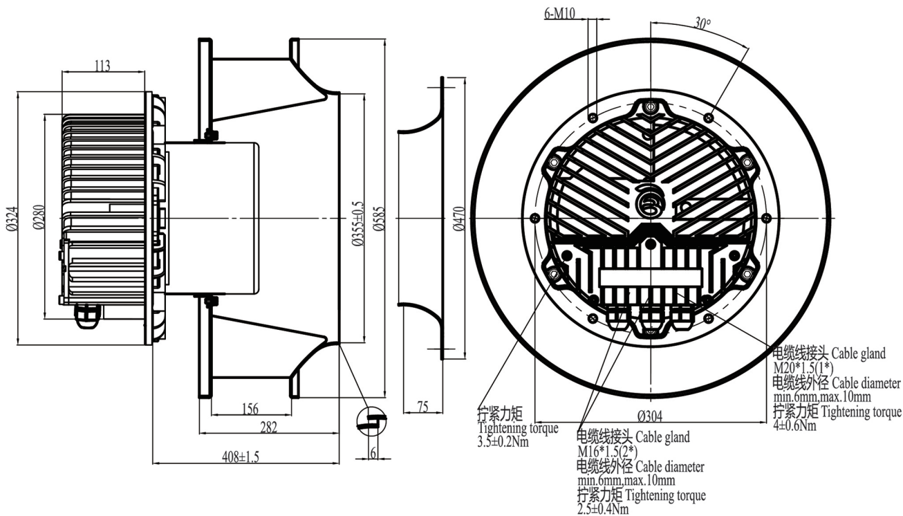
HJ6EC500/188风机整机外形图
