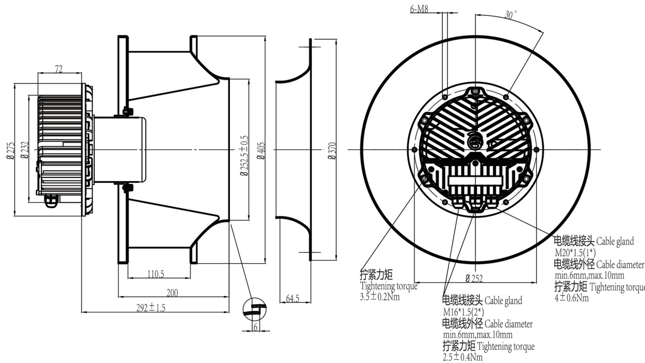
HJ6EC355/138风机整机外形图
