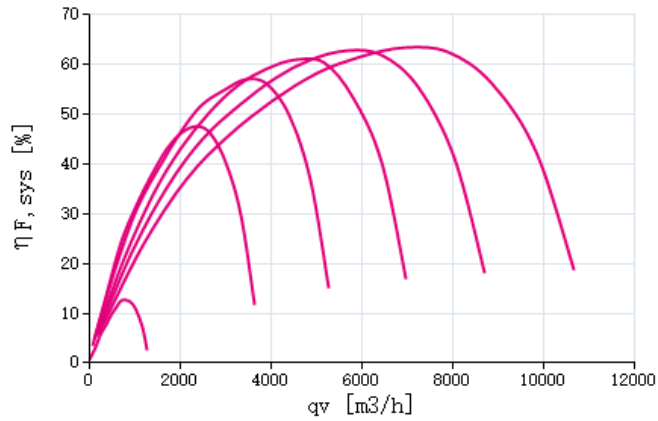
效率 \eta_{F,sys}
