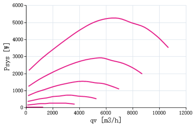
功率 P_{sys}
