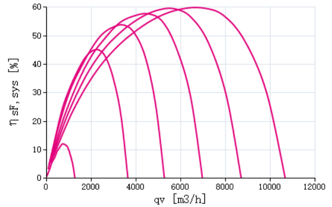
效率 \eta_{sF,sys}
